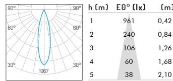
3W 24° 2700K
