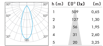
3W 36° 2700K
