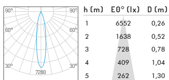
25W 15° 2700K
