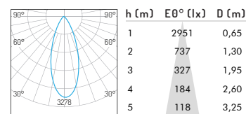
25W 36° 2700K
