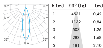
25W 24° 2700K
