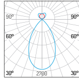
50W 50°+Batwing 3000K
