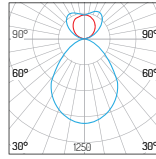
50W MPD+Batwing 3000K
